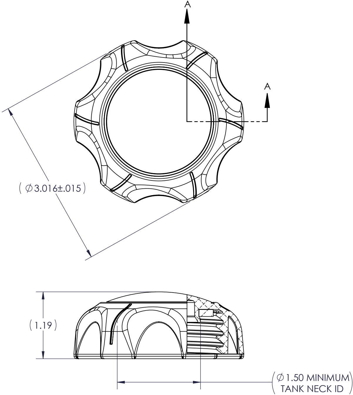
SECTION A-A
