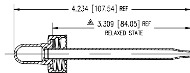
ASSEMBLED SECTION ACTUAL SIZE
