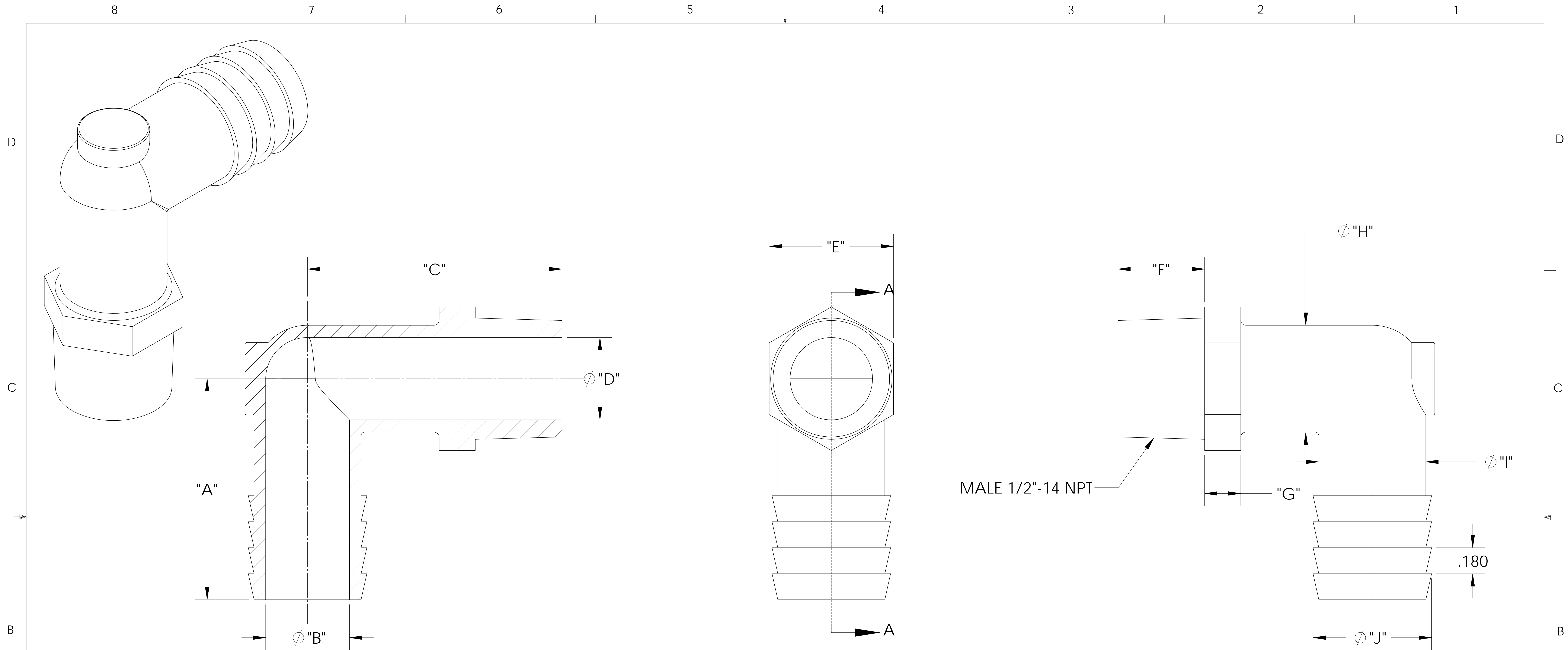
SECTION A-A
